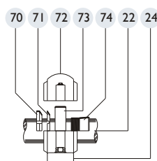
DETALHE " B " MONTAGEM DO MANCAL SN 508 (24)
