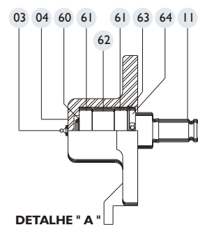
DETALHE " A " MONTAGEM DO ESTICADOR DA FITA (04)
